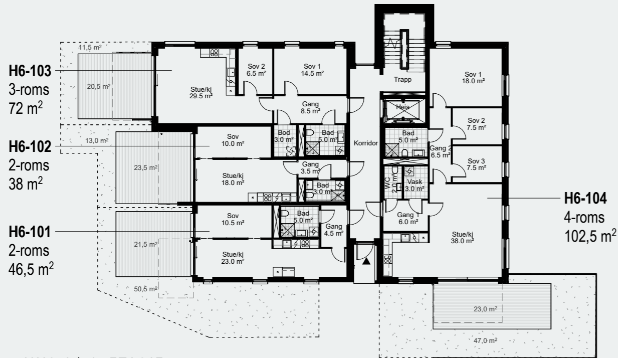
HUS 6 | 1. ETASJE
