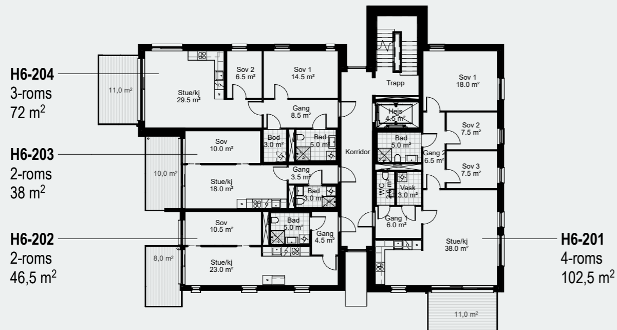
HUS 6 | 2. ETASJE
