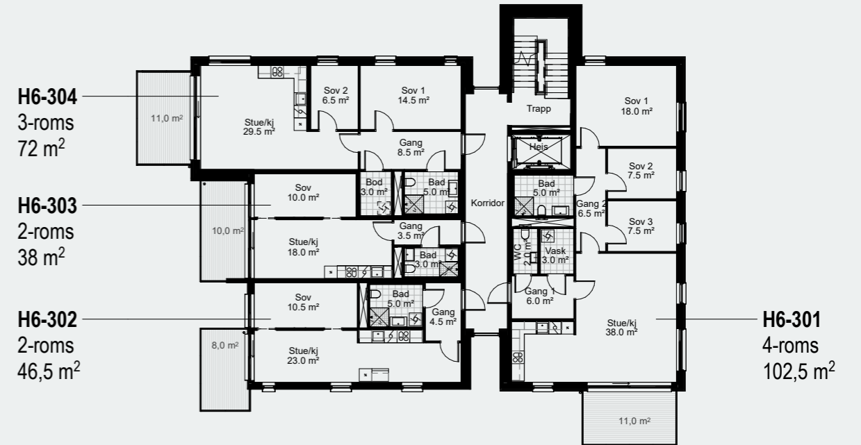
HUS 6 | 3. ETASJE
